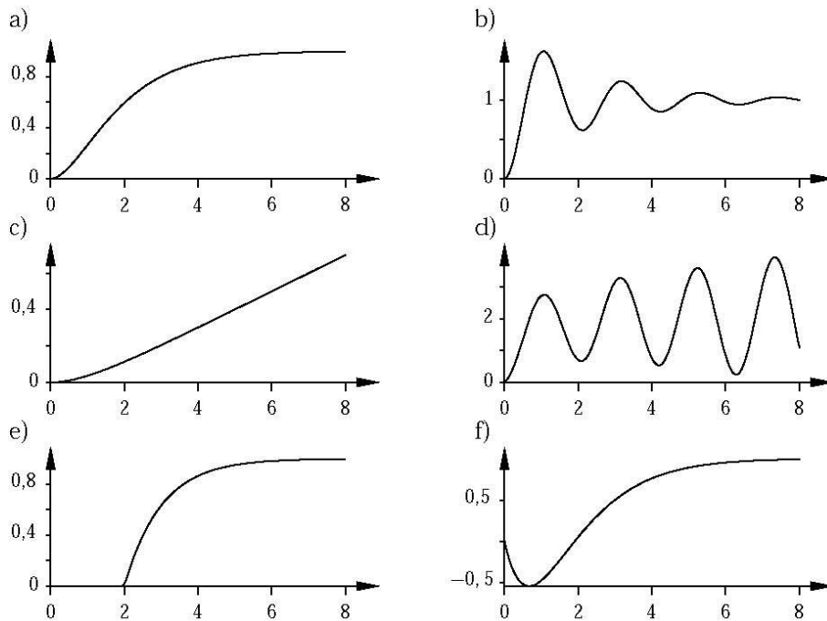
Figura 2.2 Respuestas en escalón en lazo abierto.
